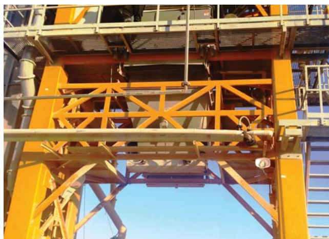
Прямая разгрузка без бункера-накопителя Direct loading, no hot mix silo
